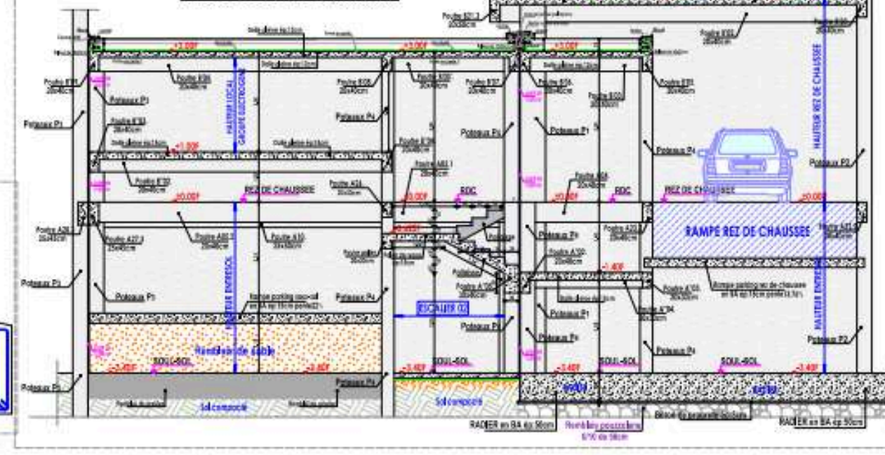
DETAIL COUPE VI-VI, Ech: 1/20e
