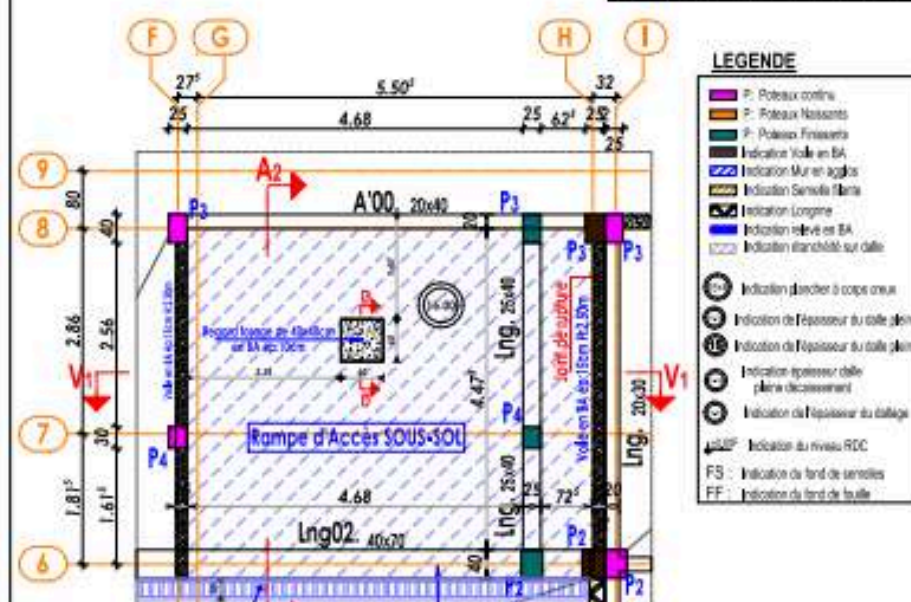
DETAIL COFFRAGE RAMPE D'ACCES SOUS-SOL
