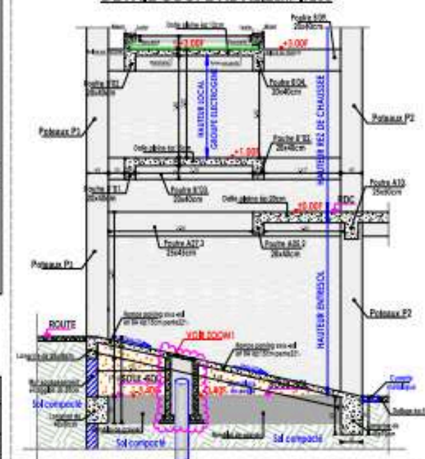
DETAIL COUPE A2-A2, Ech: 1/20e
